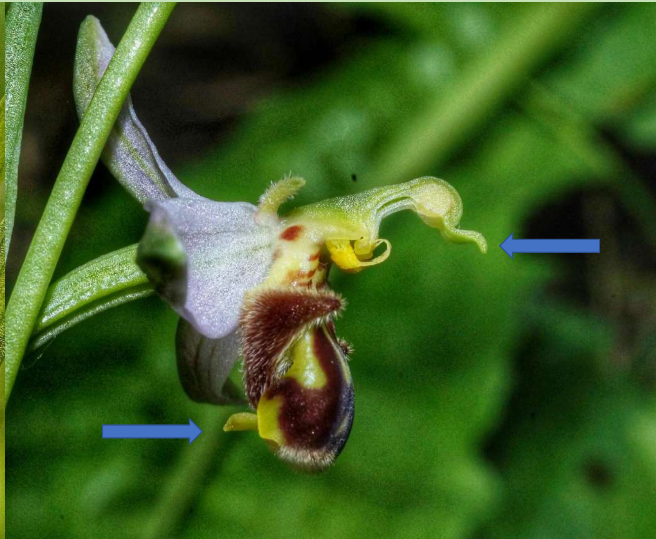
Ophrys apifera
