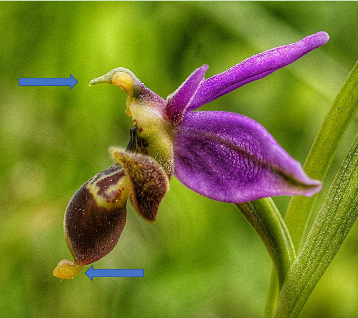
Ophrys scolopax
